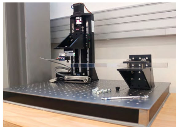
Banc de photoélasticité (plateforme génie civil)
